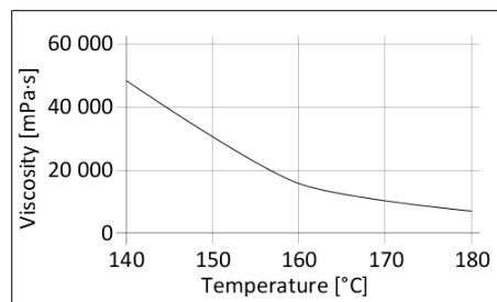
Diagram 1: Viskoznost kot funkcija temperature
