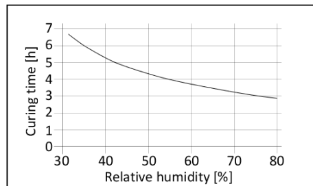
Diagram 1: Čas utrjevanja za sloj debeline 500 µm
