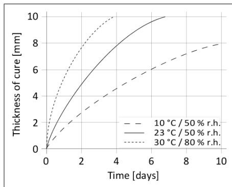
Diagram 1: Hitrost utrjevanja za SikaTack® Panel-50
