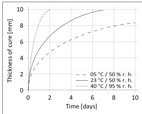
Diagram 1: Hitrost utrjevanja Sikasil® WS-300 EU
